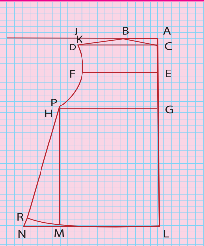
உரு 10.5 குழந்தைச் சட்டையின் பின் பகுதி
